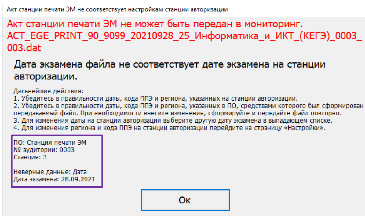
Рис. 6.30. Сообщение о несоответствии настроек в передаваемом файле акта или журнала настройкам станции авторизации (передача запрещена)
