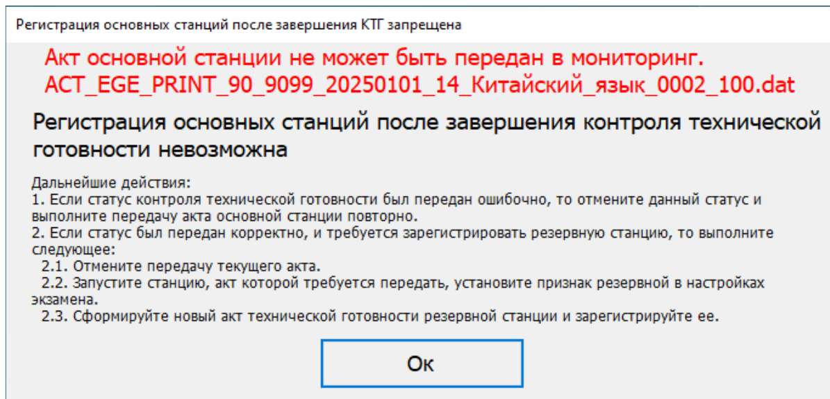
Рис. 6.36. Сообщение о запрете регистрации основных станций после передачи статуса «Контроль технической готовности завершен» (передача запрещена)
