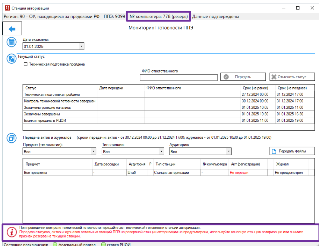
Рис. 6.4. Страница «Мониторинг готовности ППЭ». Передача статусов, актов 6 и журналов запрещены (Резервная станция)
