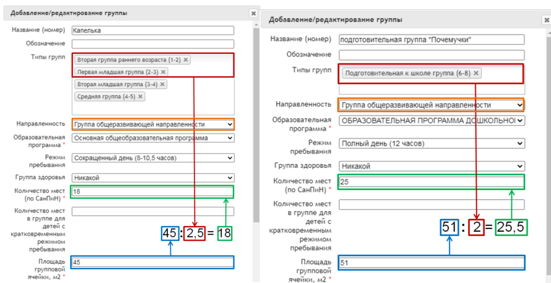
Рис. 4. Редактирование групп
